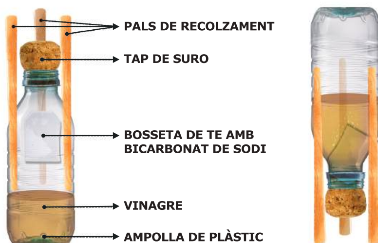
Figura 4. Muntatge experimental coet casolà
