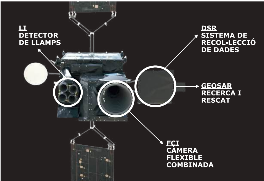
Figura 3. Animació d'un Meteosat de tercera generació Imatge extreta de: www.eumetsat.int
